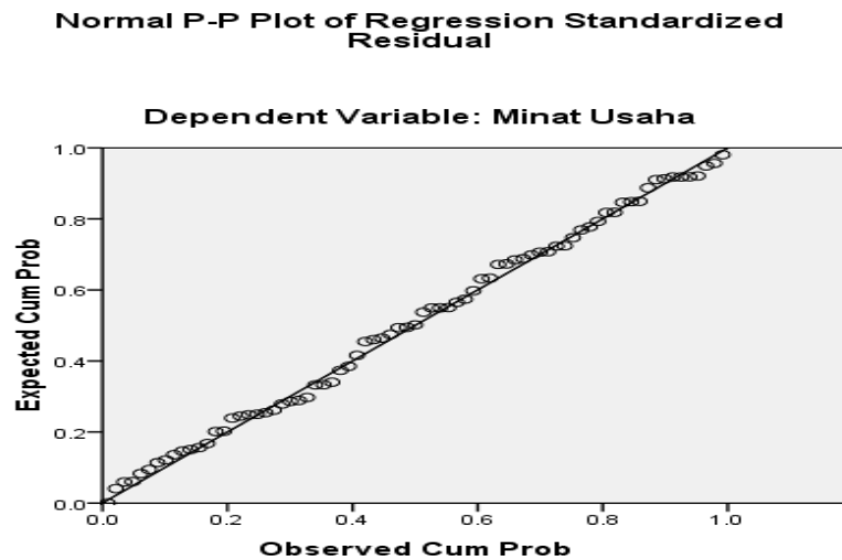
Gambar 1 Grafik Normalitas Data
