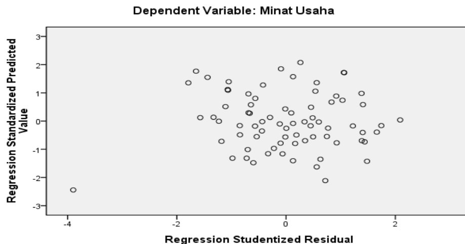
Gambar 2 Grafik Heteroskedastisitas
